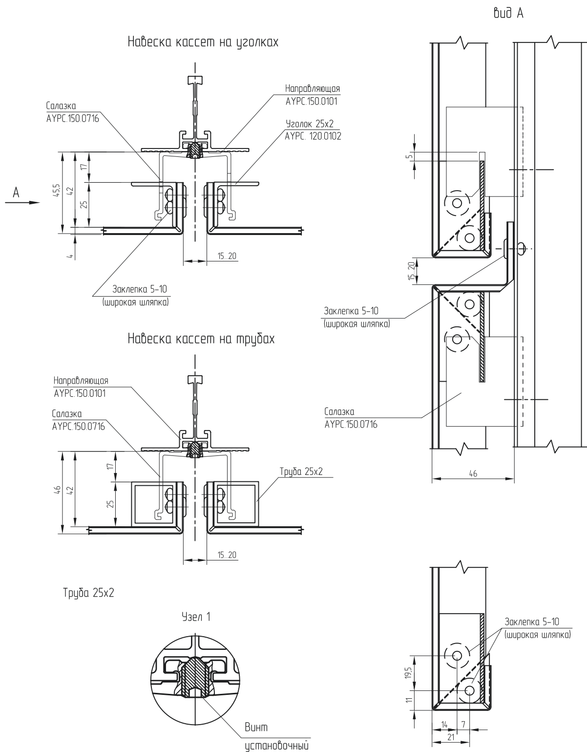
Узел 1а. Установка композитных панелей кассетного типа на салазке АУРС.150.0716. Горизонтальный разрез.
