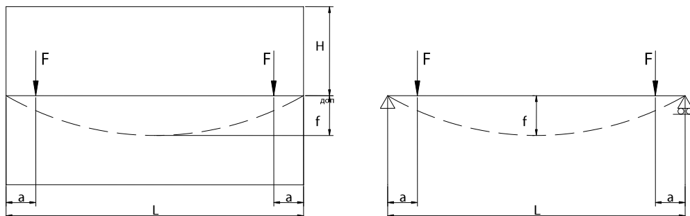
Рис. 7. Схема нагрузок
