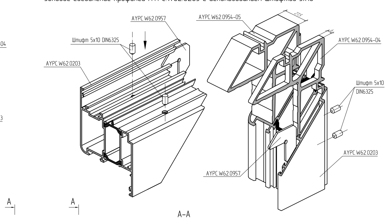
Угловое соединение профилей АУРС.W62.0203 с использованием штифтов 5x10
