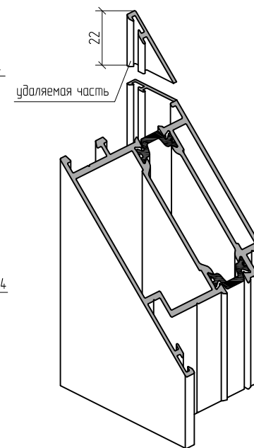
Схема обработки профиля AYPC.W62.0205
