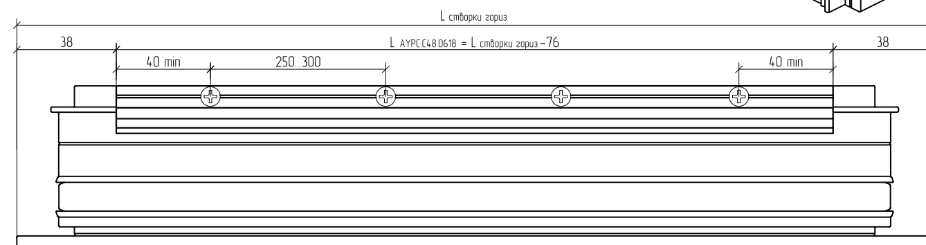
Схема установки профиля АYP C48.0618.
