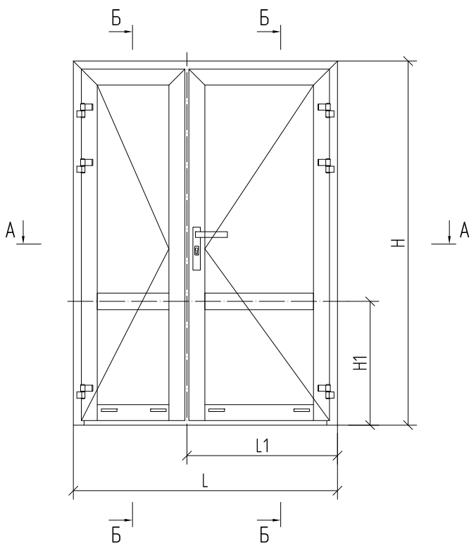
Пример расчета штапиковой двупольной двери с цоколем открыванием наружу
