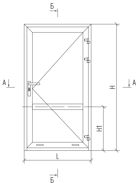
Пример расчета однопольной двери открыванием наружу
