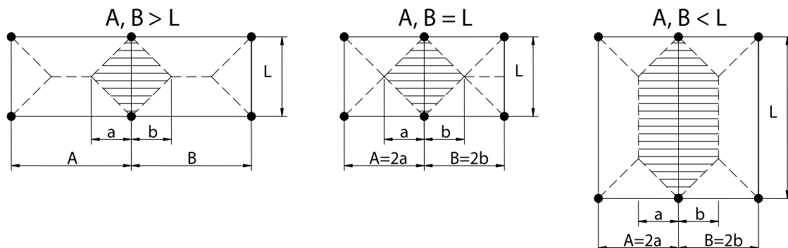
Рис. 1. Схемы нагрузок
