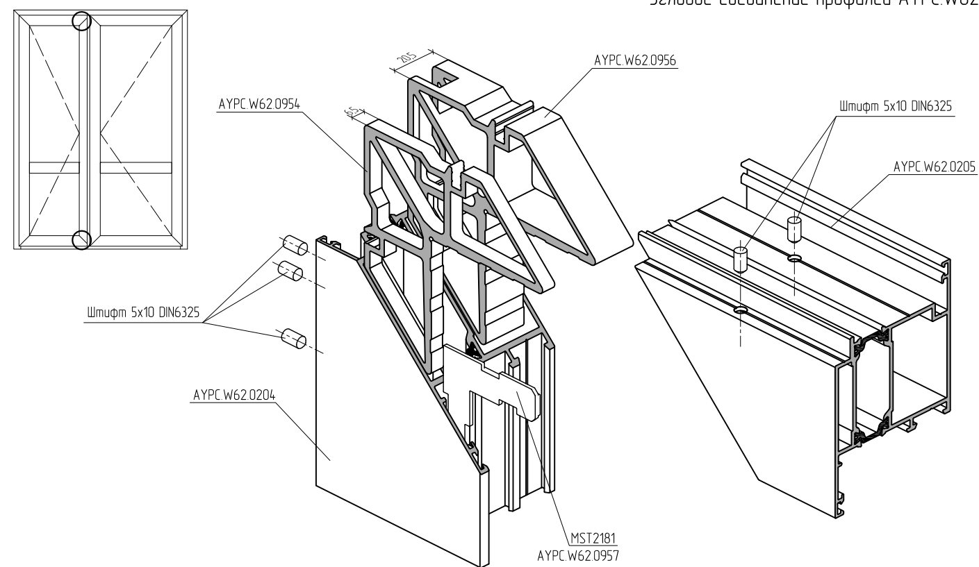
Угловое соединение профилей АУРС.W62.0205 и АУРС.W62.0204 с помощью штифтов 5х10
