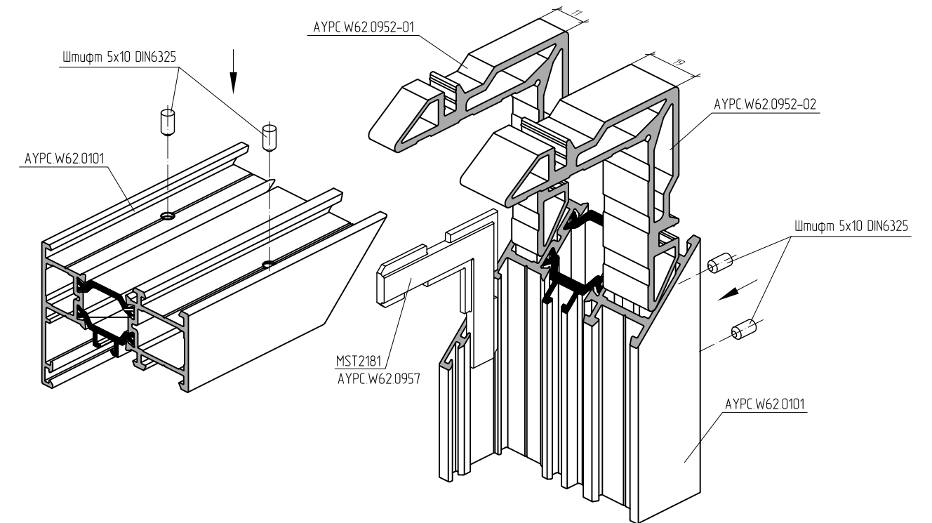
Угловое соединение профилей АУРС.W62.0101 с использованием штифтов 5x10
