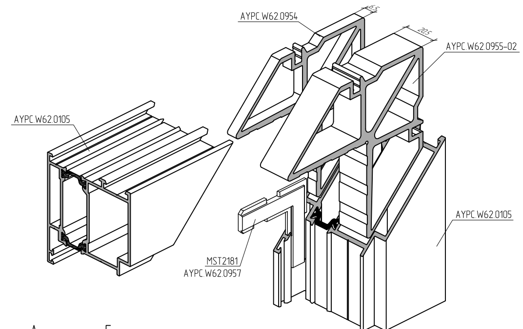
Угловое соединение профилей АУРС.W62.0105 методом обжима. Вариант 2
