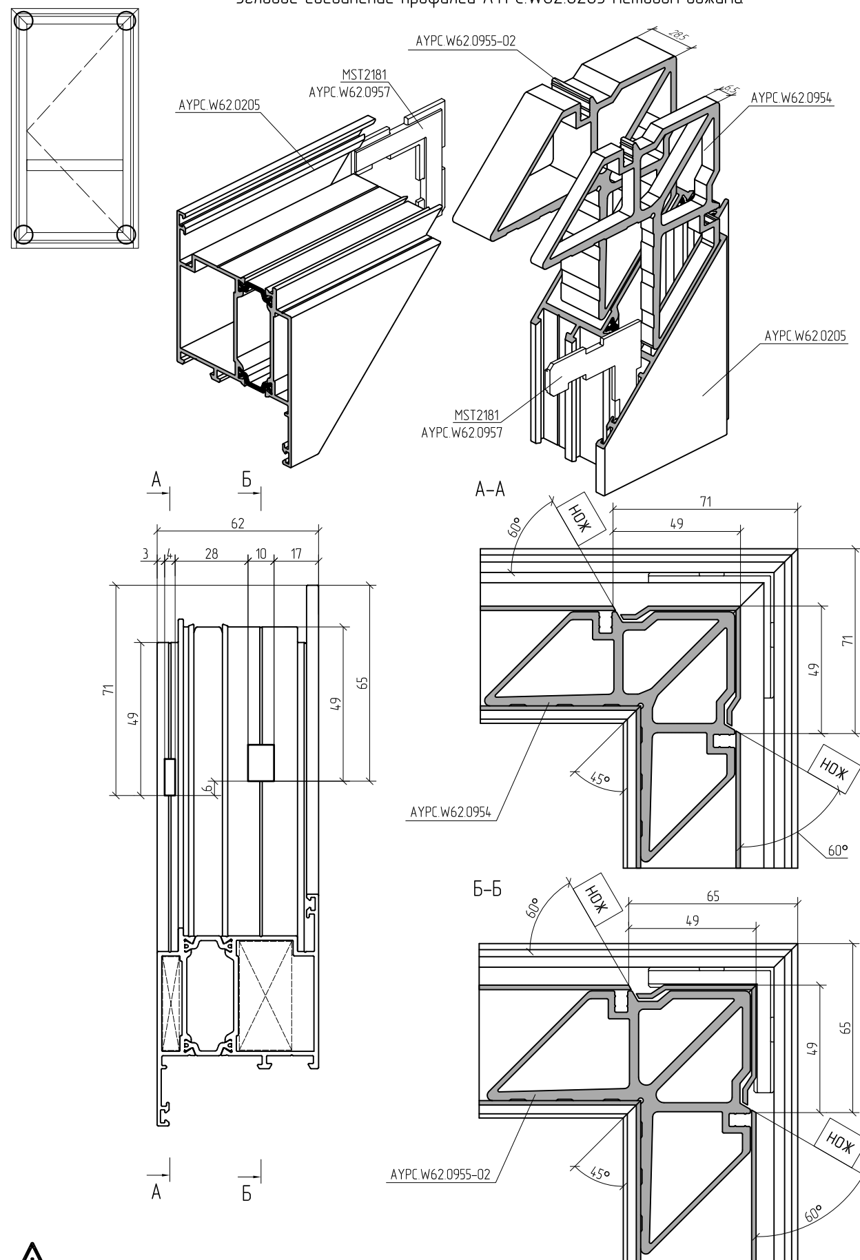
Угловое соединение профилей АУРС.W62.0205 методом обжима
