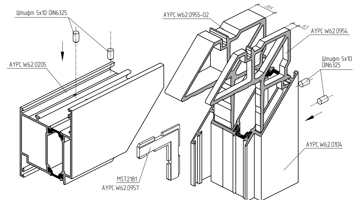
Узловое соединение профилей АУРС.W62.0104 и АУРС.W62.0205 с использованием штифтов 5х10
