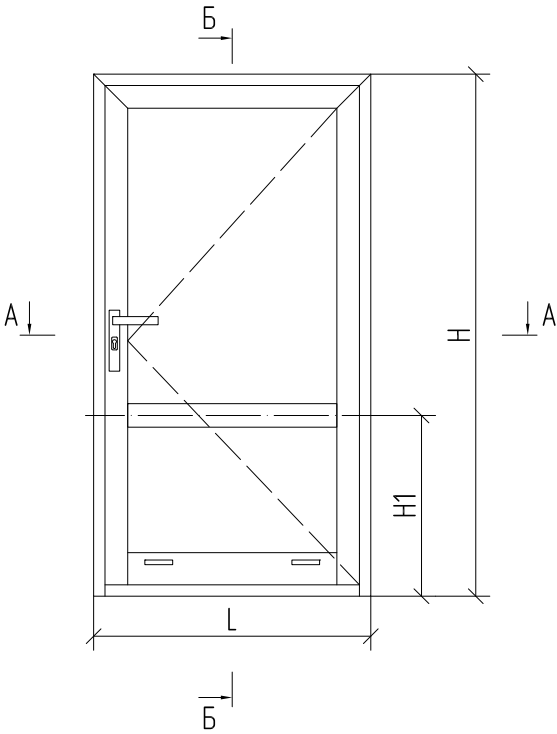
Пример расчета однополюсной двери с цоколем открыванием внутрь
